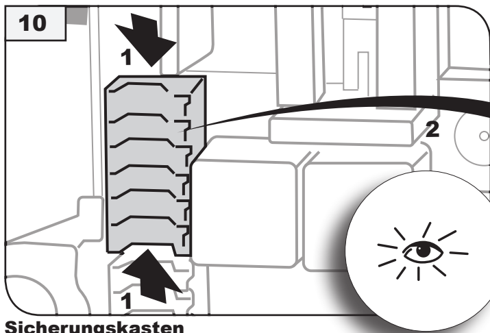
Sicherungskasten fusebox
